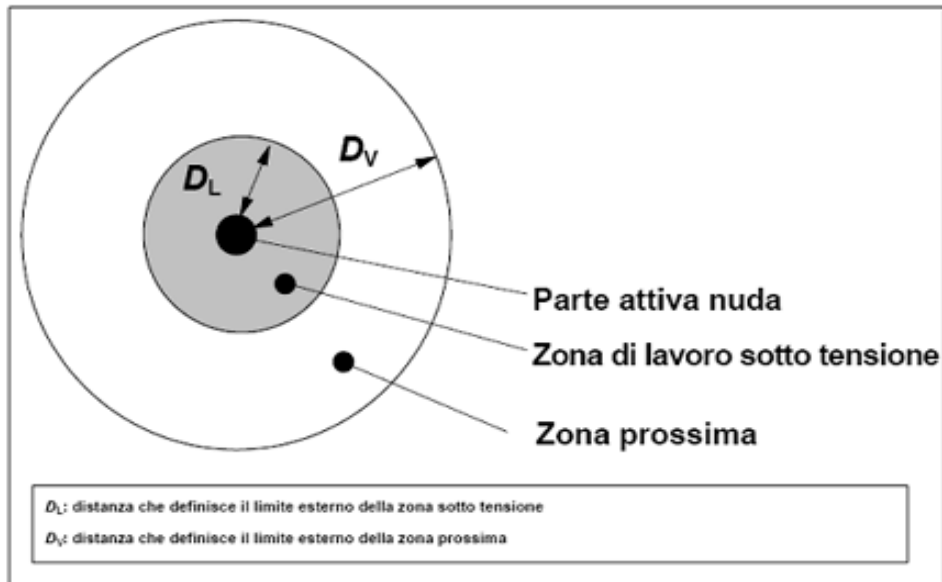
Figura 1 – Distanze in aria e zone per procedure di lavoro
